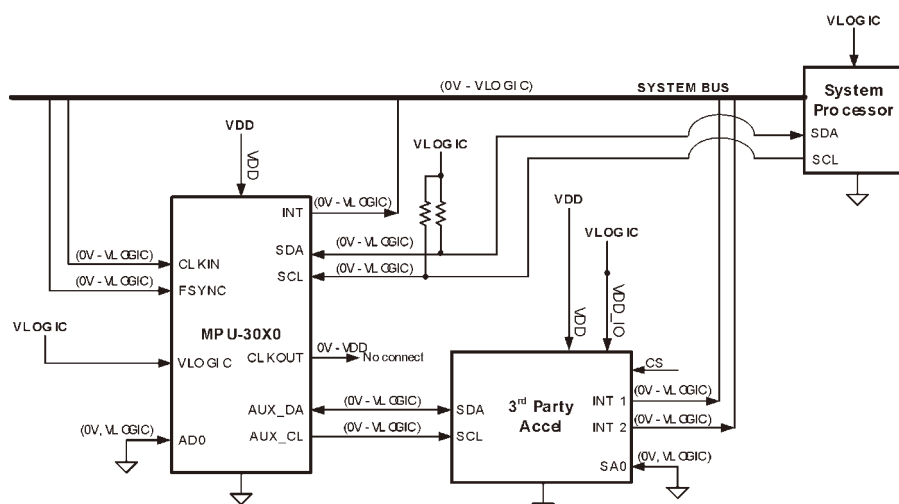
Rysunek 29. Aplikacja żyroskopu MPU-3000 lub MPU-3500
