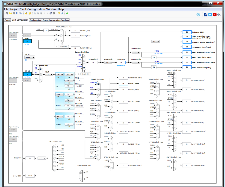
Rysunek 2. Zakładka konfiguracji taktowania
