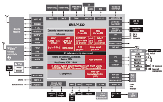
Rysunek 5. Platforma OMAP piątej generacji
