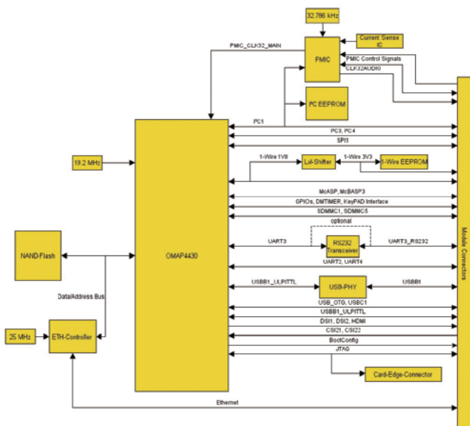
Rysunek 14. Schemat blokowy modułu firmy Phytex (OMAP 4)
