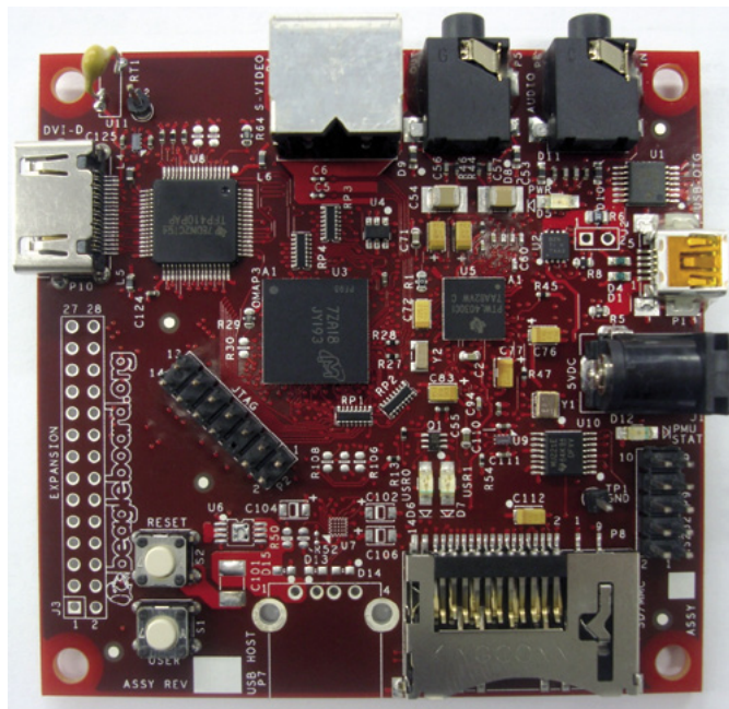
Rysunek 13. Zestaw ewaluacyjny BeagleBoard (OMAP 3)
