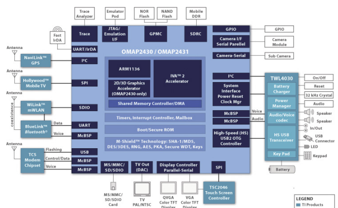
Rysunek 2. Platforma OMAP drugiej generacji
