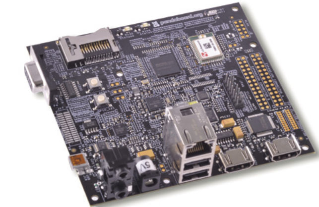
Rysunek 12. Zestaw ewaluacyjny PandaBoard (OMAP 4)
