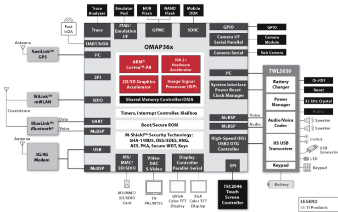
Rysunek 3. Platforma OMAP trzeciej generacji
