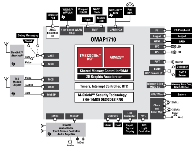
Rysunek 1. Platforma OMAP pierwszej generacji
