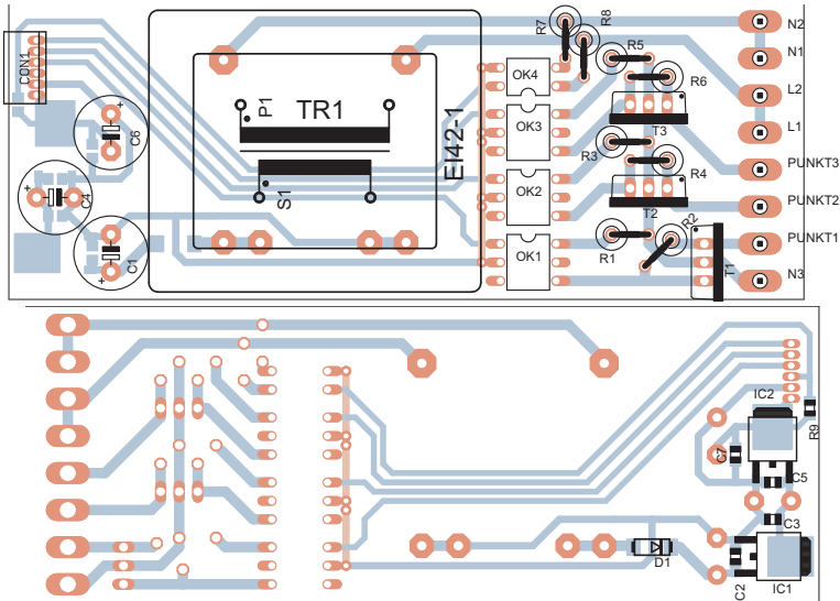
Rysunek 7. Schemat montażowy modułu sterującego-zasilającego
