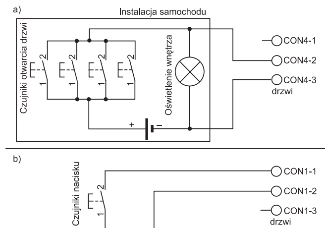
Rys. 2. Warianty podłączenia do instalacji samochodu a) podłączenie do instalacji oświetlenia wnętrza pojazdu; b) podłączenie własnego czujnika
